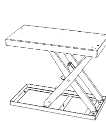
Einfach-Scherensystem
